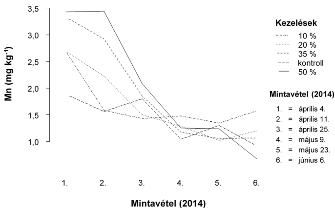
3. ábra: A tápközeg minták 0,01 M \text{CaCl}_2 -os Mn-tartalma
